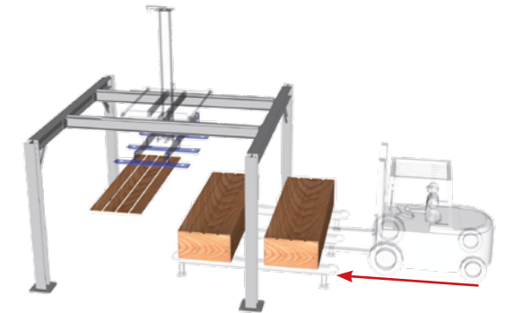
A. Breites Gestell für frontale Zufuhr mit dem Stapler.
