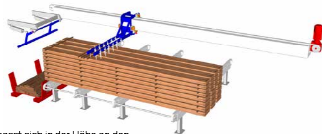
B. Die Kehrvorrichtung passt sich in der Höhe an den Stapel an.
