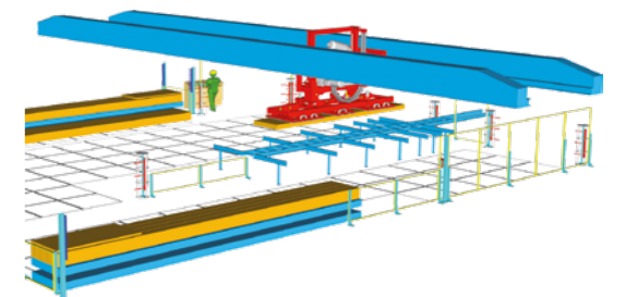
D. Y horizontale Bewegung mit Kran und Laufkatze.
