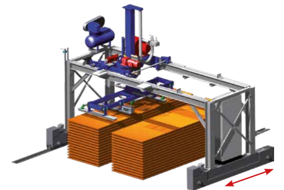
C. Y horizontale Bewegung mit zwei fahrbaren Einheiten.
